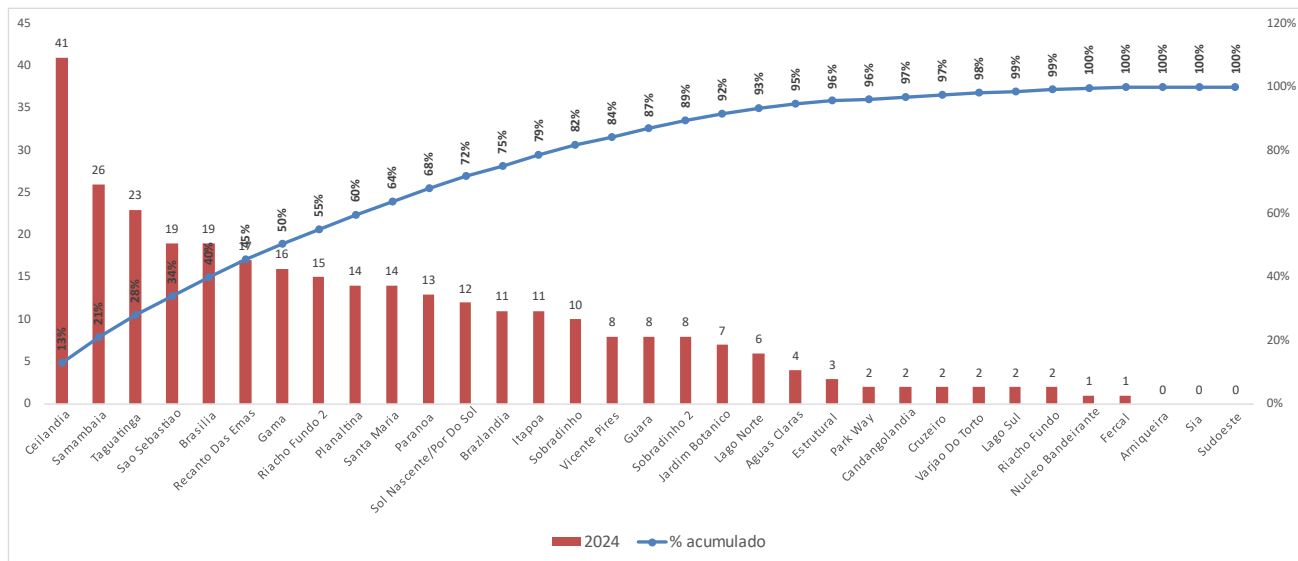
Gráfico 1 – Gráfico de Pareto da Participação percentual – Ano 2024.
